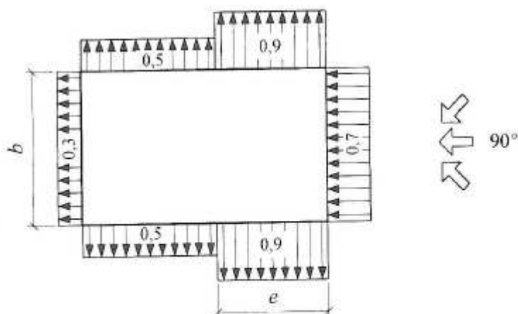
Figur V 6.3.1.1 – Formfaktorer c_{pe,10} for ydervægge vist på grundplan
