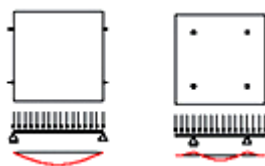
Fig. 18 Principskitse af traditionelle ophængningsystemer med dorne (t.v.) i forhold til ACT, hvor bøjningsmomentet er reduceret (t.h.) [Fischer 2006].
